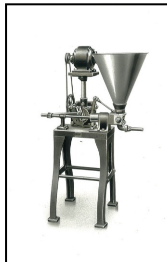
Remplisseuse de pommade
