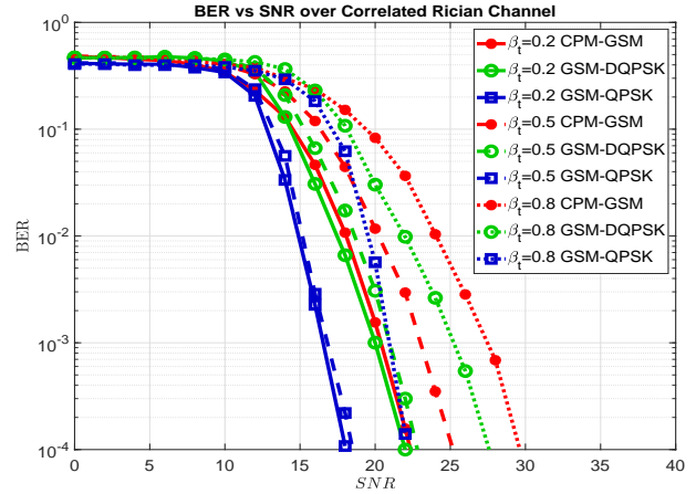
FIGURE 3 – TEB vs SNR pour (D)QPSK-GSM et CPM-GSM sur canal de Rice corrélé
