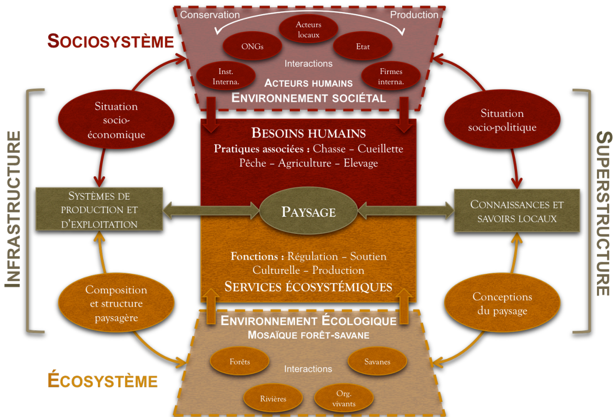
Figure 1 : Système complexe développé à partir des concepts de socio-écosystème et de formation socio-spatiale plaçant le paysage au centre des interactions humains-milieu, adapté aux caractéristiques sociales et écologiques de la zone étudiée (réalisation Christophe Demichelis).
