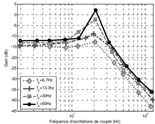
Fig. 5. Diagrammes de gain mesurés pour plusieurs fréquences d'alimentation
