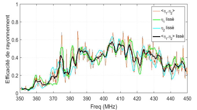
Figure 9. Efficacité de rayonnement moyenne comparée aux efficacités propres à chaque antenne (configuration chaotique).
