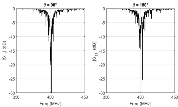
Figure 3. S_{11} mesuré en Chambre Réverbérante pour deux positions différentes du brasseur.
