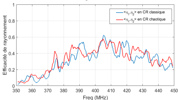
Figure 11. Efficacité de rayonnement moyenne calculée dans les deux configurations de la CR.
