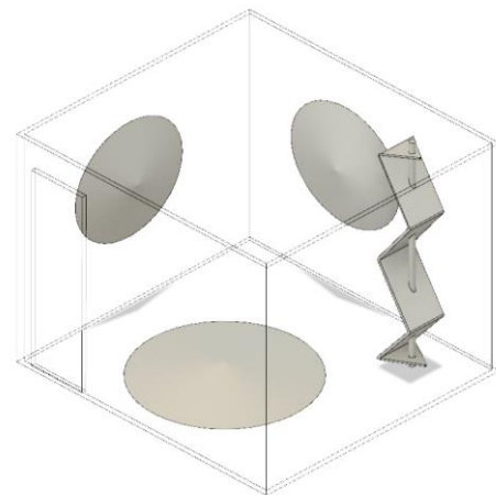
Figure 1. Chambre réverbérante du laboratoire ESYCOM munie de trois calottes sphériques.
