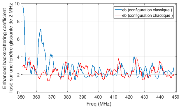
Figure 10. Coefficient de rétrodiffusion ' eb ' dans les deux configurations de la CR.
