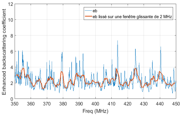
Figure 6. Coefficient de rétrodiffusion 'eb' de la chambre réverbérante.
