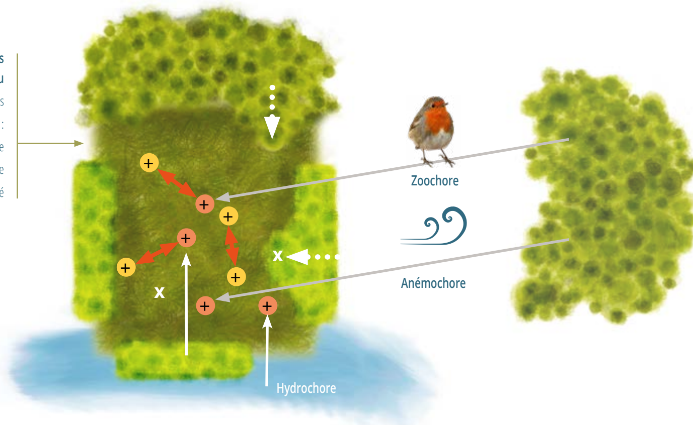
Figure 4.2 : Schéma bilan des paramètres et processus impliqués dans la succession végétale, FMA, 2018.
