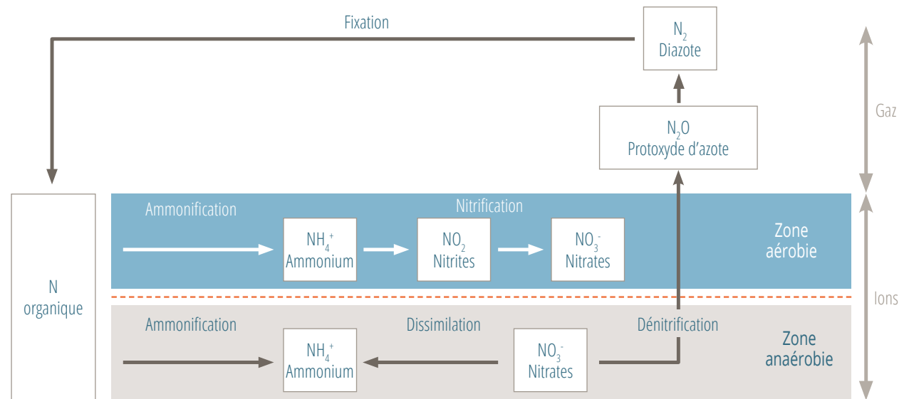
Figure 6.6 : Cycle de l'azote simplifié en zone humide d'après REDDY et PATRICK, 1984 in CLEMENT, 2001
