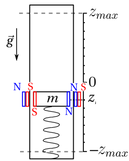
(d) With HSLD stiffness
