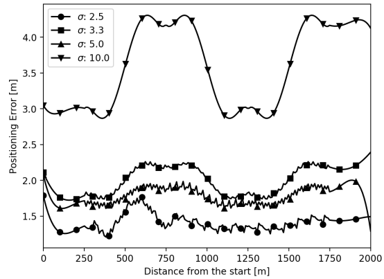
FIGURE 2: Erreur de positionnement
