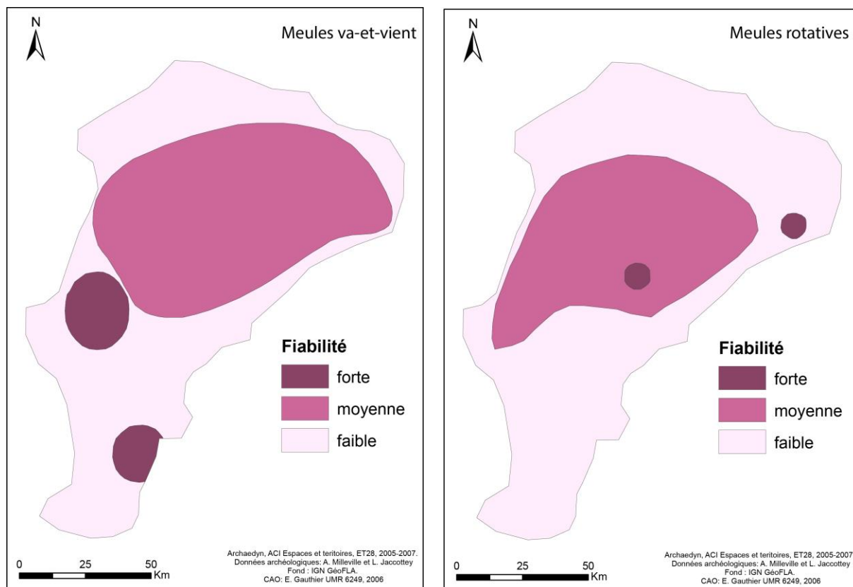
Fig. 11. Carte de fiabilité de la répartition du matériel de mouture en Franche-Comté. A gauche : meules va-et-vient, à droite : meules rotatives (Données : A. Milleville et L. Jaccottey, CAO : E. Gauthier, 2006).
