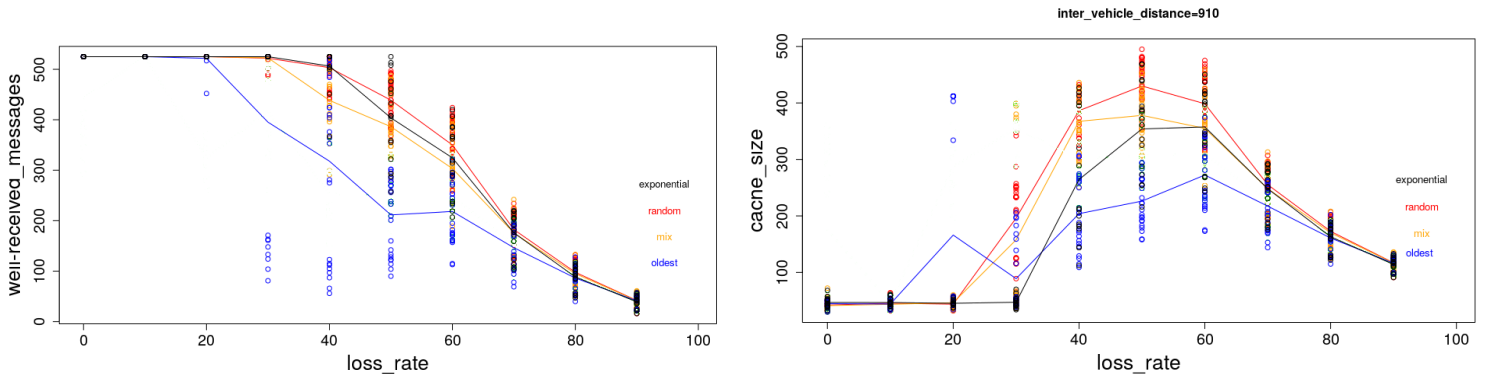
FIGURE 1: Métriques d'efficacité applicative \mathbf{ae} (gauche) et de consommation de ressources \mathbf{rm} (droite) en fonction du taux de perte
