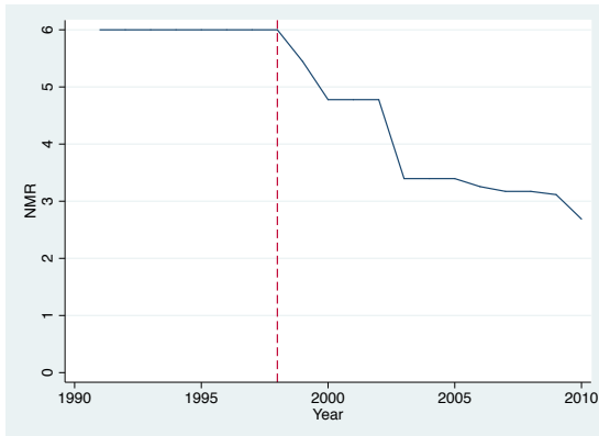
Portugal: NMR
