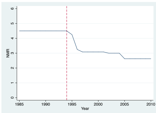
Austria: NMR
