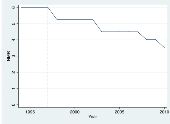
Finland: NMR
