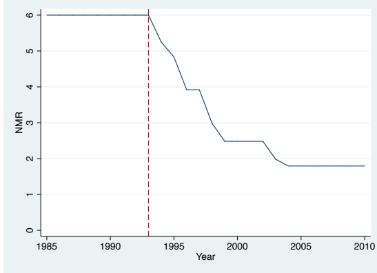
Canada: NMR
