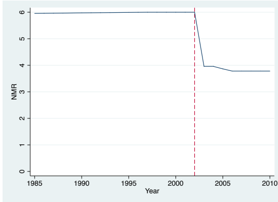
Ireland: NMR
