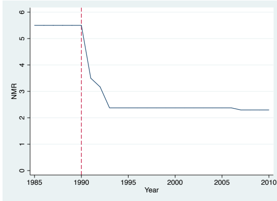
Poland: NMR
