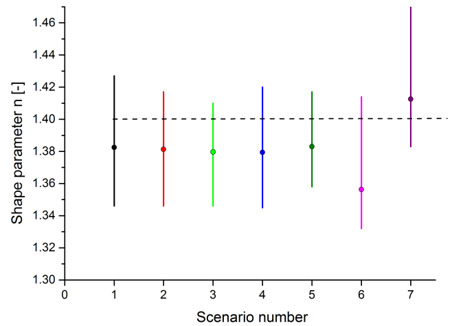
Figure 13. Posterior mean values and 95 % confidence intervals of the shape parameter n for the different scenarios.
