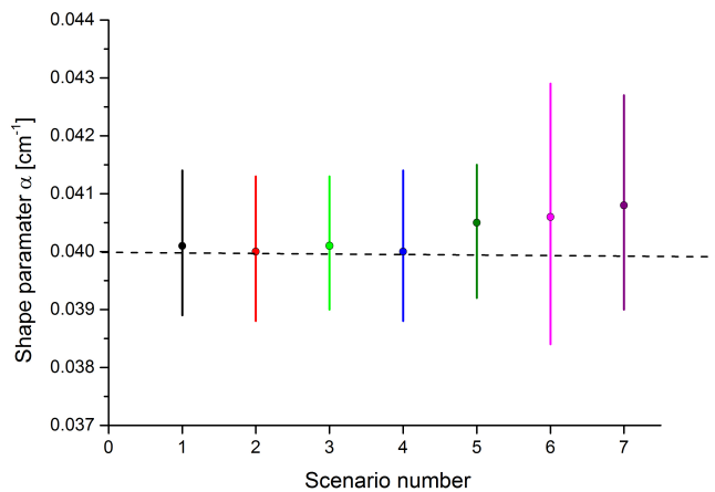
Figure 12. Posterior mean values and 95 % confidence intervals of the shape parameter \alpha for the different scenarios.
