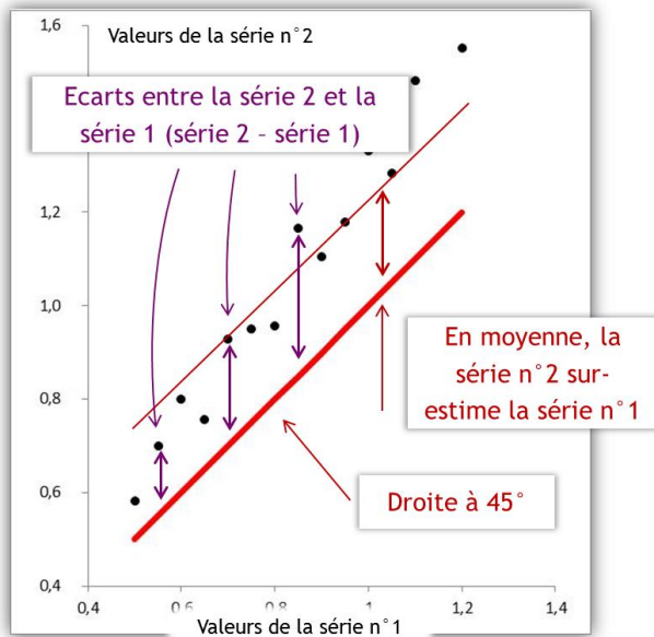
Figure 5. Illustration de deux critères de concordance dans la méthode de Bland et Altman : l'écart moyen entre la série de mesures n°2 et la série de mesures n°1 (écart entre la droite rouge en trait fin et la droite à 45°), et l'ensemble des écarts entre les deux séries de mesures.
