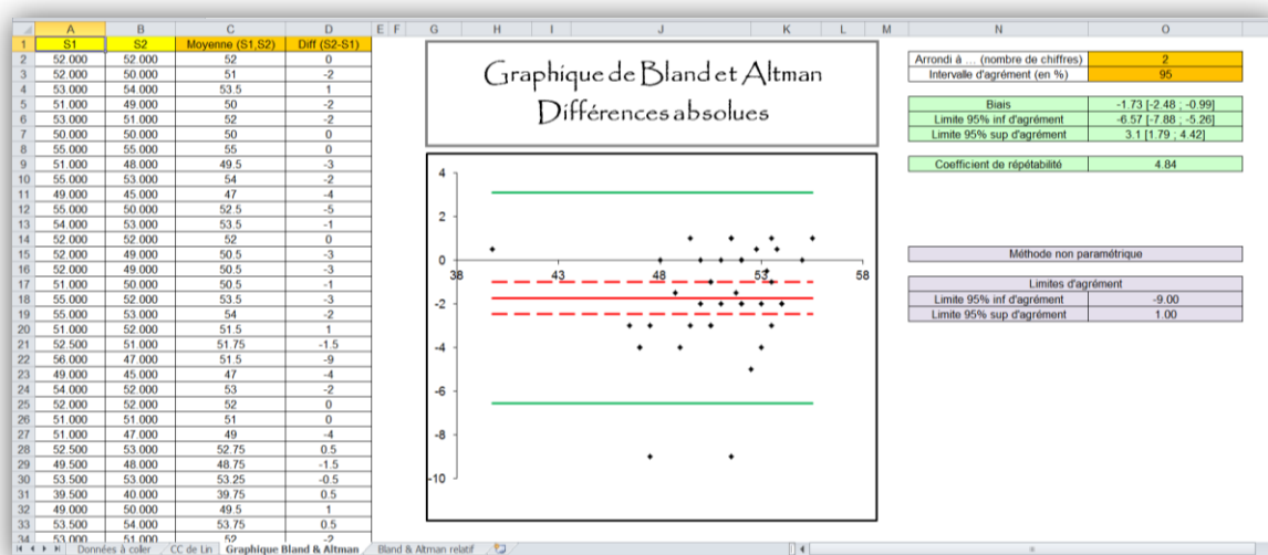
Figure 10. Graphique de Bland et Altman représentant la concordance des mesures de HCC entre celles effectuées par CB et celles effectuées par MH.
