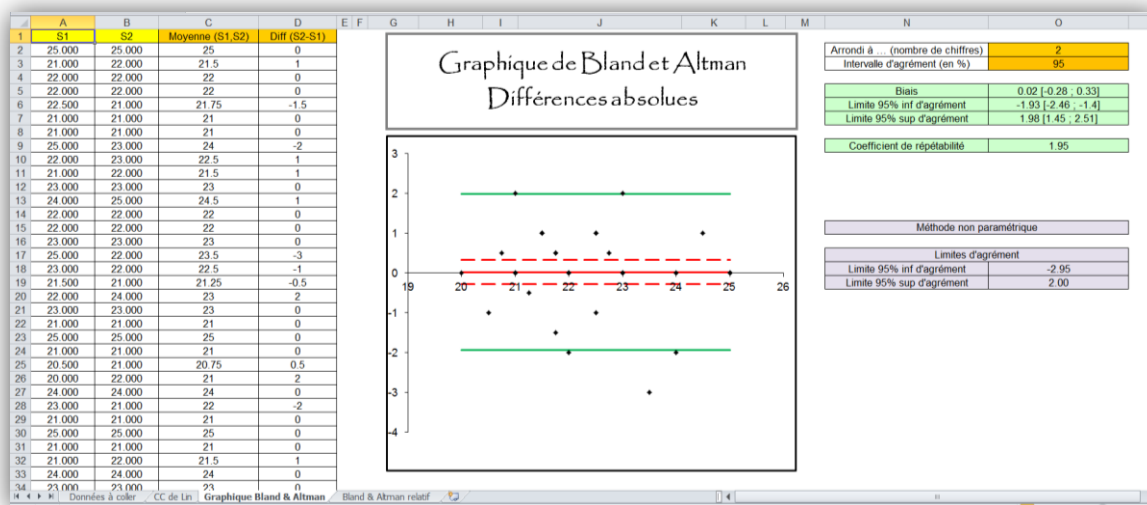
Figure 9. Graphique de Bland et Altman représentant la concordance des mesures de HDV entre celles effectuées par CB et celles effectuées par MH.
