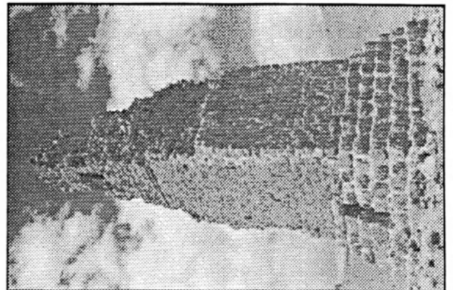
La tour d'Atenatan (n°7) à Palmyre (9 av. J.-C.) Vue du sud-est ; plans du rez-de-chaussée et du 1er étage.
