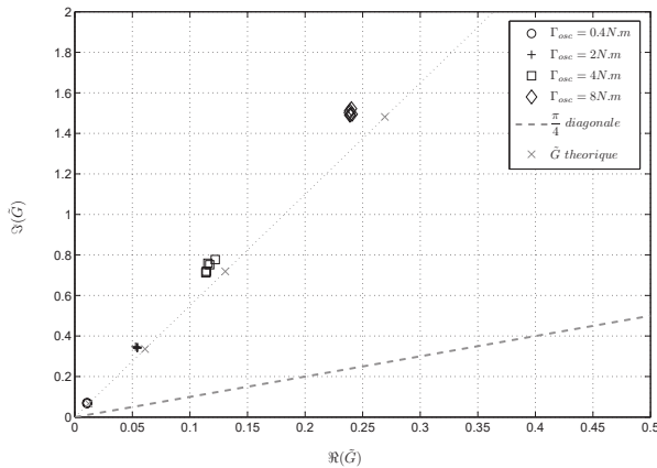
Fig. 4. Vecteur complexe \tilde{G} en cas d'oscillations du couple de charge - Résultats théoriques et résultats expérimentaux pour f_{osc} = 120Hz
