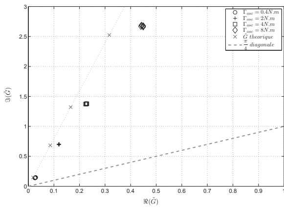
Fig. 3. Vecteur complexe \tilde{G} en cas d'oscillations du couple de charge - Résultats théoriques et résultats expérimentaux pour f_{osc} = 20Hz
