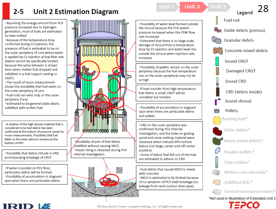
Figure 2: Schéma estimatif de la nature et du positionnement des débris attendus sur la tranche 2 (au 3/7/2017 [11])
