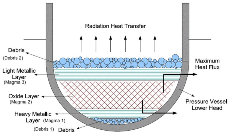
Figure 1: Configuration typique du corium en fond de cuve (tiré de [9])
