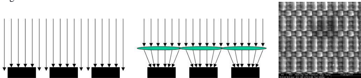
Figure 6 – Effet des microlentilles pour un capteur à transfert interligne, et vue au MEB pour un capteur réel (source EMA)
