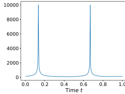
(d) Intermediate gradient iterations: case 2
