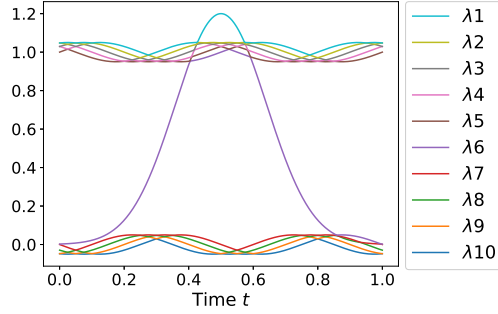
(a) Reordered eigenvalues \lambda_i(t)
