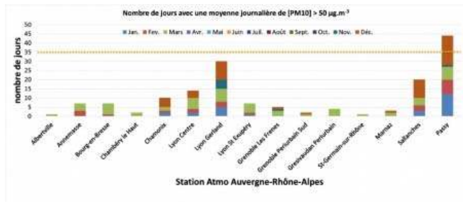
Figure 2. Nombre de jours sur l'année 2015 dépassant le seuil des 50 \mu\text{g}/\text{m}^3 de concentration moyenne journalière en \text{PM}_{10} sur plusieurs sites de mesure Atmo Auvergne-Rhône-Alpes de la région Rhône-Alpes. Le détail de la contribution de chaque mois est donné par un code couleur. Le trait tireté horizontal orange marque le seuil réglementaire de 35 jours par an de dépassement, défini par l'article R221-1 du code de l'environnement (source : Atmo Auvergne-Rhône-Alpes).
