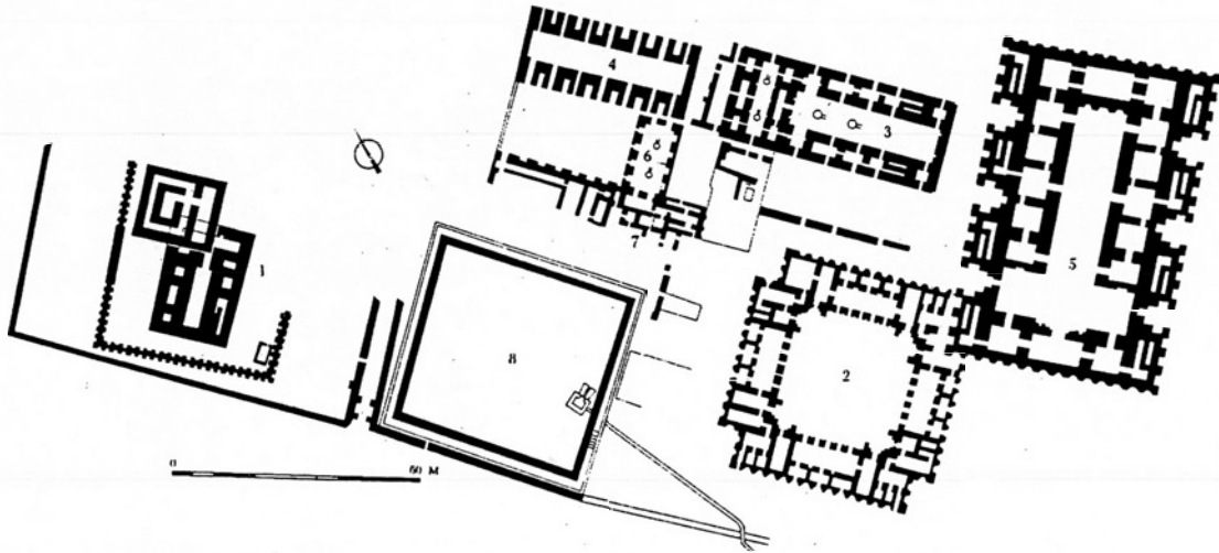
Fig. 1. Uruk. Constructions du secteur de l'E.ANNA, niveaux VI-IV (fin IV e millénaire av. J.-C.) Dessin Giroux, d'après H. Lenzen dans P. Amiet, L'art antique du Proche-Orient , Paris, 1977, p. 526.
