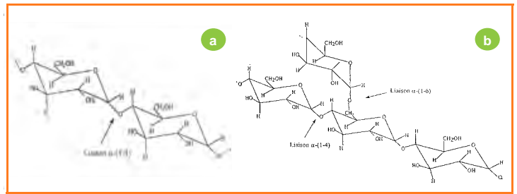
Figure 12 - Structure chimique de l'amylose (a) et de l'amylopectine (b).
