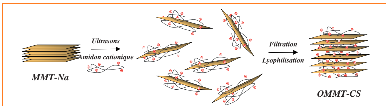
Figure 24 - Représentation schématique de la modification de la montmorillonite en présence d'amidon cationique.
