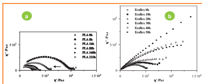
Figure 26 - Évolution de la viscoélasticité à l'état fondu (diagrammes de Cole-Cole) après photovieillement accéléré pendant des durées variables : (a) poly(acide lactique) ; (b) copolyester poly(butylène adipate-co-téréphtalate) [29].
