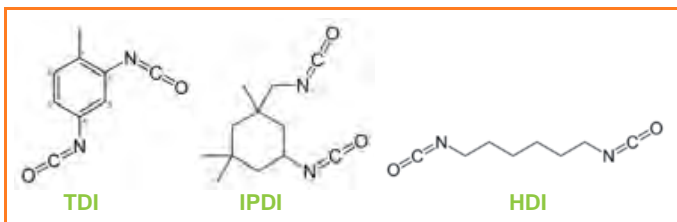
Figure 11 - Formules chimiques du toluène diisocyanate (TDI), de l'isophorone diisocyanate (IPDI) et de l'hexaméthylène diisocyanate (HDI).
