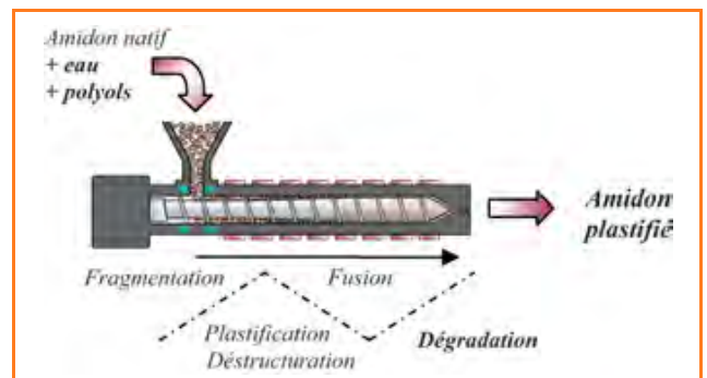
Figure 13 - Représentation schématique de l'extrusion de l'amidon plastifié.
