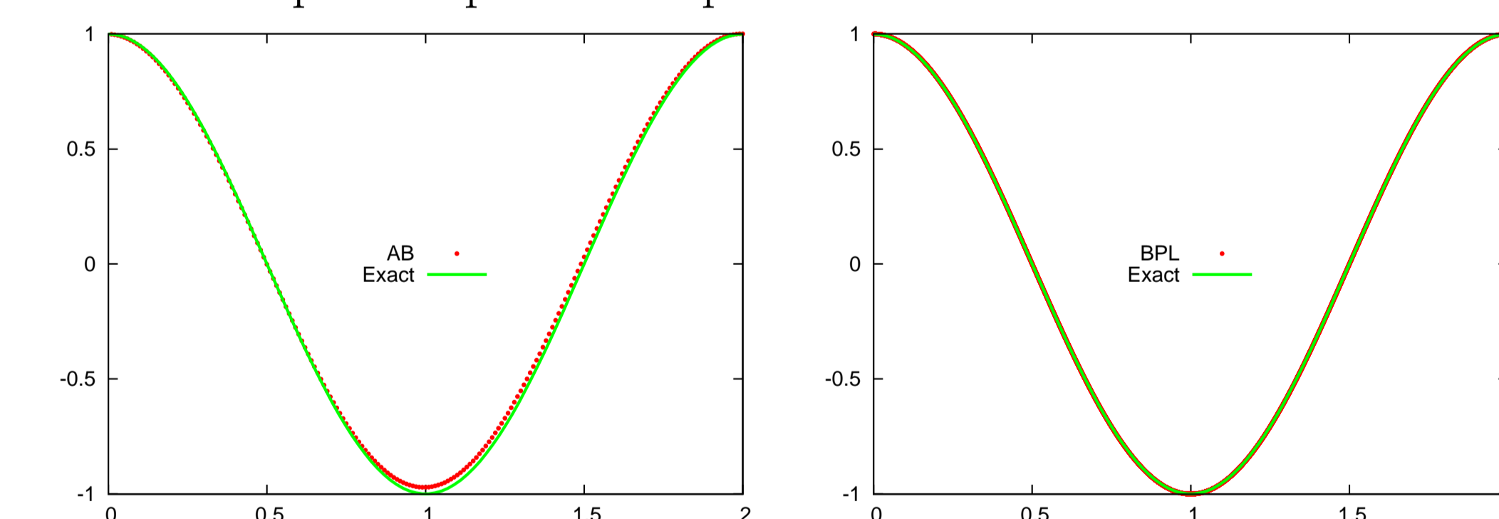
AB = Adams-Bashforth. BPL = Décomposition en série + resommation
