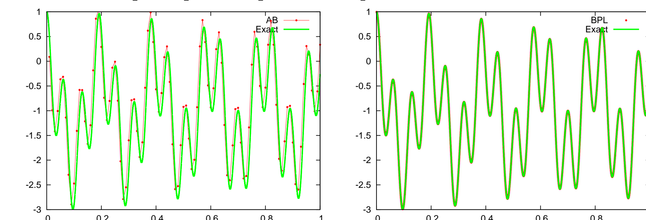
AB = Adams-Bashforth. BPL = Décomposition en série + resommation
