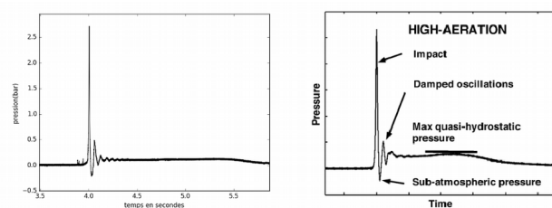
Figure 4 : à gauche signal de pression mesuré sur la digue de l'Artha le 4 avril 2016 à 15h. À droite schéma d'un impact haute aération selon [7]
