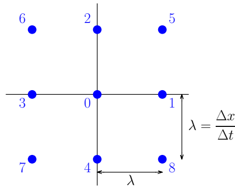
Figure 1: D2Q9
