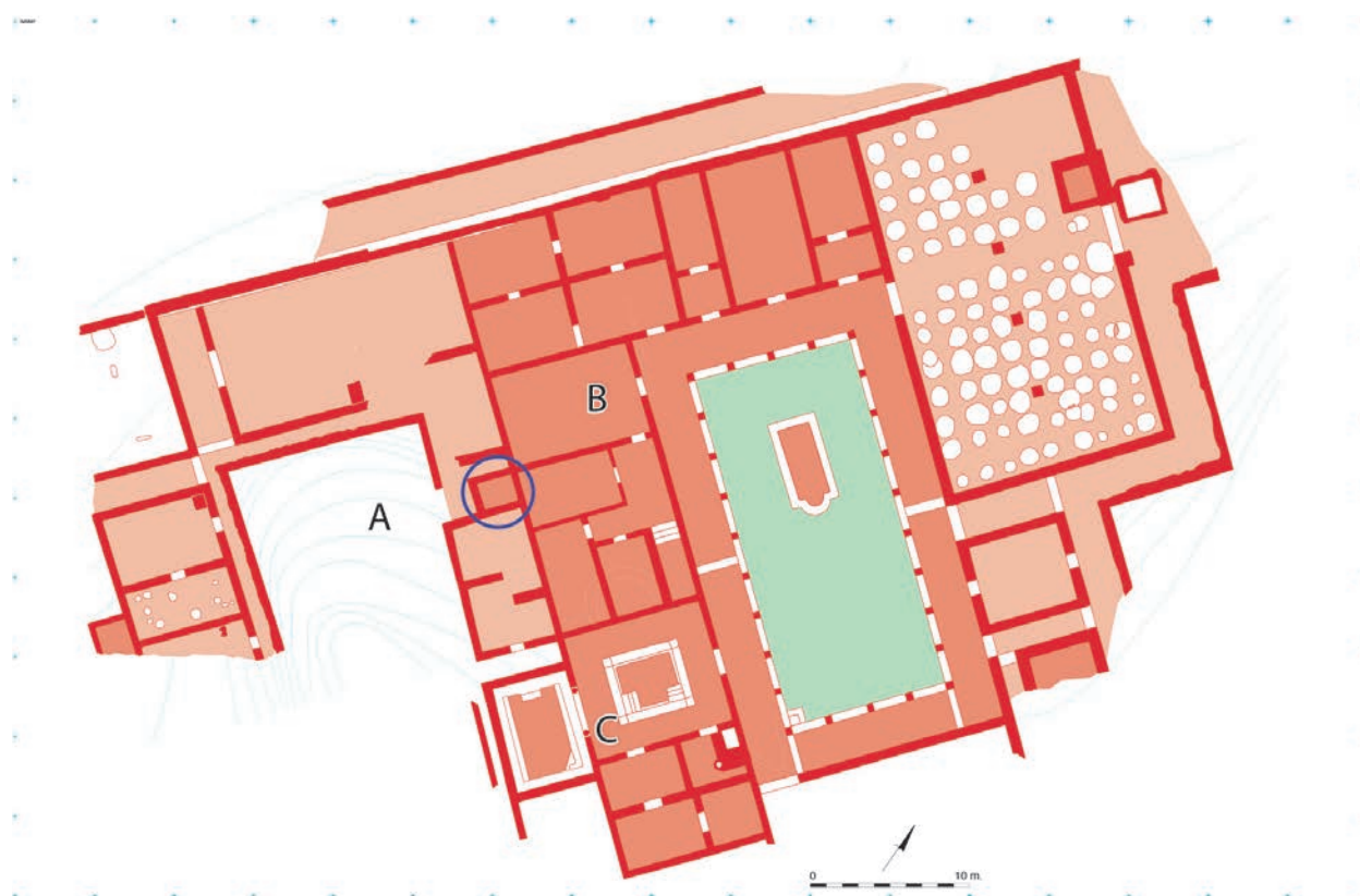
Figure 2. La villa du Haut-Empire et la localisation du chauffage par convection. A, cour secondaire, logements des dépendants ; B, aile occidentale de la résidence ; C, bains.
