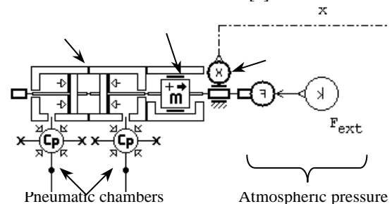
Fig. 5 Pneumatic jack model in AMESim.
