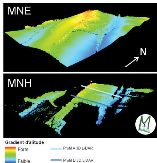
Figure 3 ci-dessous - Vue 3D du rectangle d'emprise du MNE (en haut) et MNH (en bas) représentant la topographie de la canopée du bois de La Broquière sous le logiciel LP360, fonctionnant dans l'environnement ArcGis. Le logo représente la mission d'acquisition couplée de données LiDAR et hyperspectrale par capteurs aéroportés (projet MADONNA) réalisée en juillet 2010 financée par l'INRA et l'INP.
