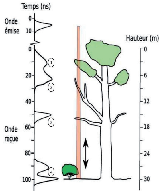
Figure 1 - Ondes laser émises et reçues sur une zone de végétation complexe. Tous les objets suffisamment résolus spatialement contribuent à la forme de l'onde via le retour des 4 échos : 1 : premier retour, 2 et 3 : retours intermédiaires et 4 : dernier retour.
