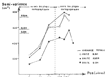
Figure 3 : Variogramme de la profondeur du sol. Variogram of soil depth.
