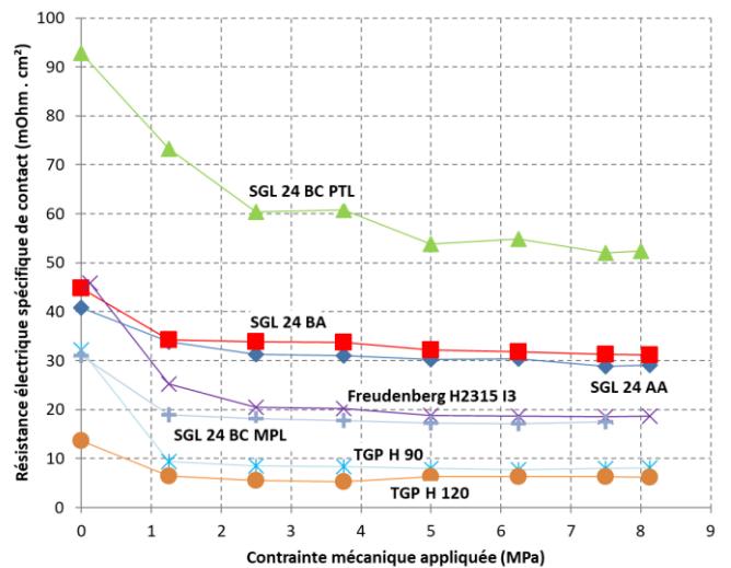
Fig. 5. Résistances électriques de contact entre la GDL et la plaque bipolaire en fonction de la contraite mécanique pour les sept références de GDLs étudiées (mesure réalisée après 5 cycles de compression).
