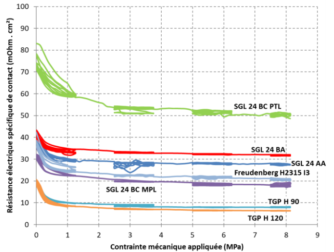
Fig. 4. Résistances électriques de contact entre la GDL et la plaque bipolaire en fonction de la contraite mécanique pour les sept références de GDLs étudiées (cas de l'essai 3).
