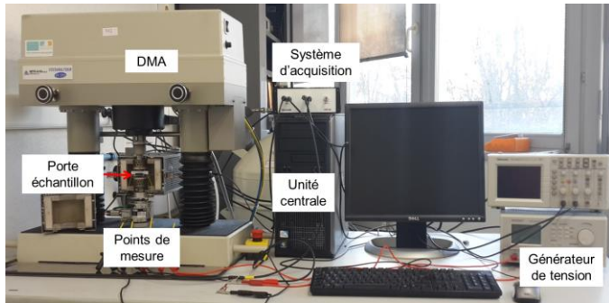
Fig. 1: Montage expérimental.
