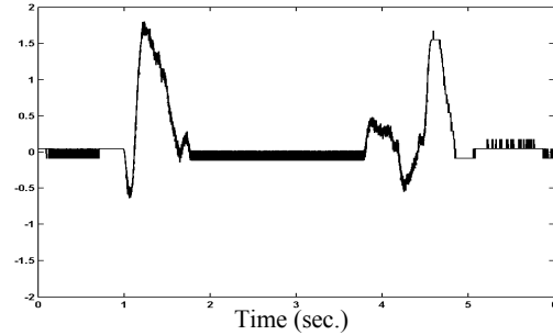
Fig. 8. Position error (mm)
