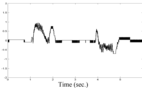
Fig.11. Position error (mm)
