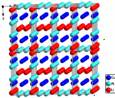
Fig. 1. Illustration de la structure T_1 vue dans le plan a-c proposée par Donnadiu [2].
