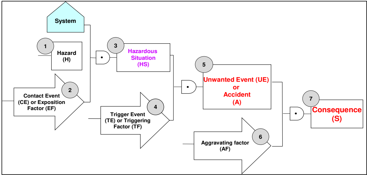
Fig 1. Accident scenario (Desroches, 2013).
