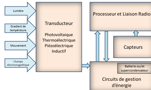
FIGURE 1 – Schéma d'un noeud de capteur autonome
