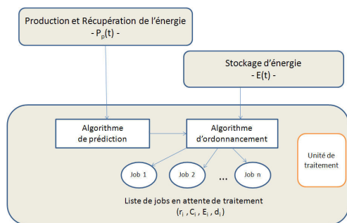
FIGURE 2 – L'ordonnanceur temps réel
