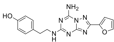
ZM-241385
