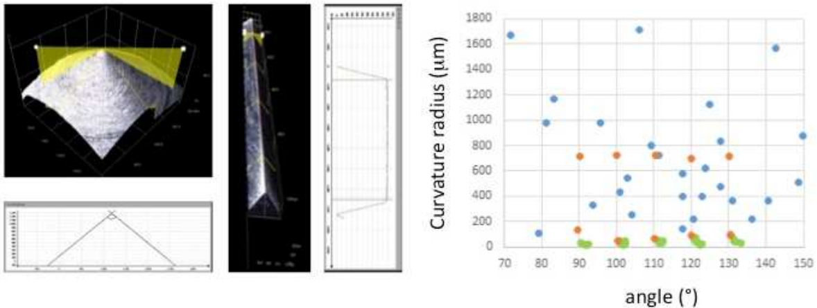
Figure 6 : Les formes géométriques des indentateurs dimensionnés pour l'étude (points rouges pour les indentateurs coniques et les points verts pour des indentateurs en forme de dièdre). Les points bleus sont des mesures de la surface inférieure de la couche d'enrobé indentant la grille.
