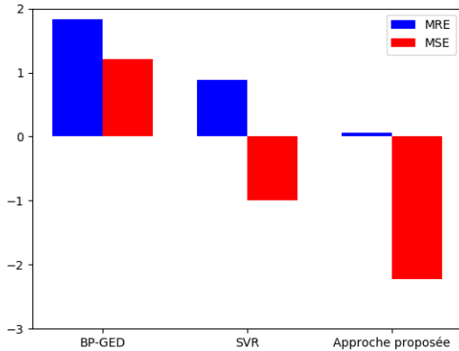
FIGURE 10 – Résultats obtenus par les méthodes BP-GED, SVR et notre méthode sur la base FINGERPRINT en MRE et MSE. Le \log_{10} des résultats est utilisé pour une meilleure lisibilité.
