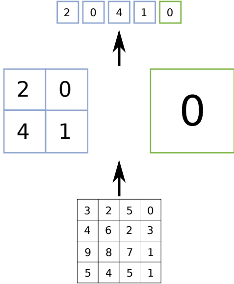
FIGURE 5 – Spatial Pyramid Pooling appliqué à une matrice 4 \times 4 pour des N de valeur 1 et 2.
