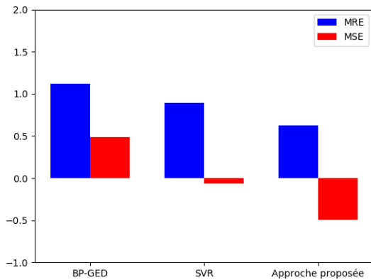
FIGURE 8 – Résultats obtenus par les méthodes BP-GED, SVR et notre méthode sur la base LETTER en MRE et MSE. Le \log_{10} des résultats est utilisé pour une meilleure lisibilité.
