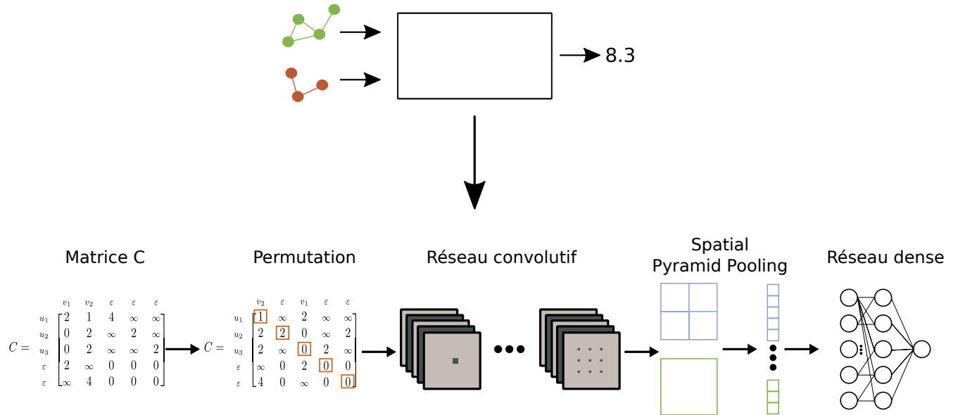
FIGURE 6 – Processus final de la méthode.
