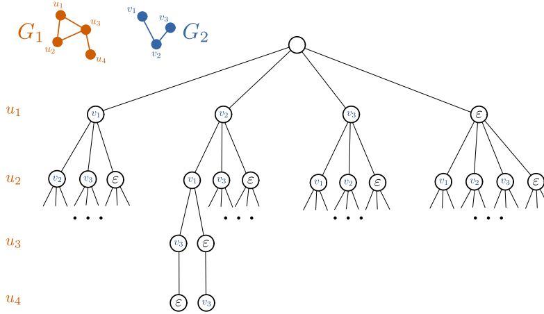
FIGURE 1 – Arbre partiel représentant l’ensemble des chemins d’édition entre G_1 et G_2 . L’algorithme A^* permet de parcourir cet arbre afin de trouver un chemin de coût minimal.
