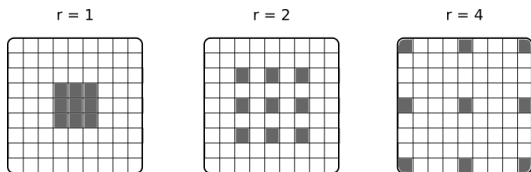
FIGURE 4 – Représentation visuelle des convolutions dilatées.
