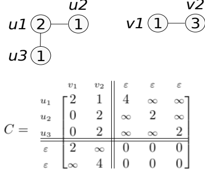
FIGURE 2 – Exemple de matrice de coût pour deux graphes. Les nœuds du graphes sont attribués. Le coût de substituer deux nœuds correspond à la différence entre leurs attributs. Le coût de substituer deux arcs est nul. Les coûts d'insertions/suppressions des nœuds/arcs valent 1.
