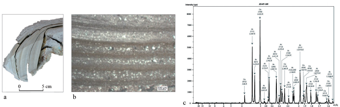
Fig. 7. Le faciès A des travertins des thermes de Jebel Oust (mission Jebel Oust, J. Curie). a. Observation à l'échelle macroscopique ; b. Lecture microscopique ; c. Diffractogramme de résultat de l'analyse DRX (Ca. = calcite ; Ar. = aragonite).
