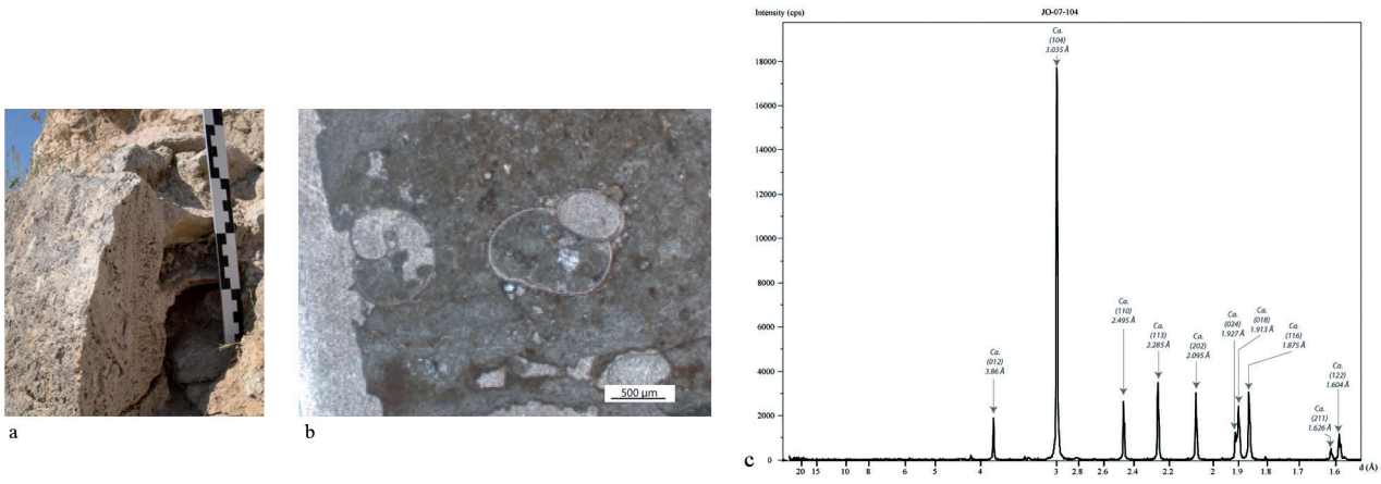
Fig. 9. Le faciès C des travertins des thermes de Jebel Oust (mission Jebel Oust, J. Curie). a. Observation à l'échelle macroscopique ; b. Lecture microscopique ; c. Diffractogramme de résultat de l'analyse DRX (Ca. = calcite).
