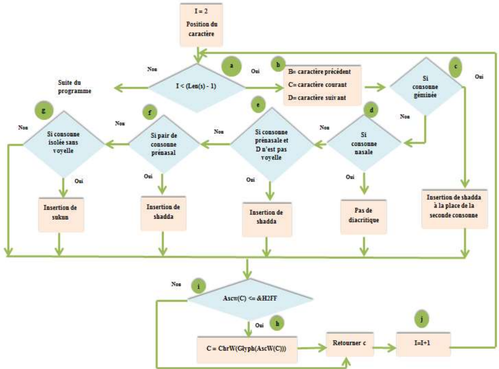
Figure 5: Organigramme de la translittération des consonnes
