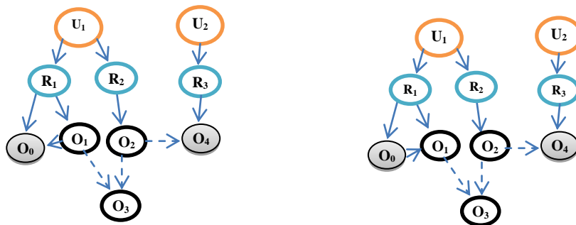
Figure 4 Règle d'inférence par un intermédiaire non autorisé
