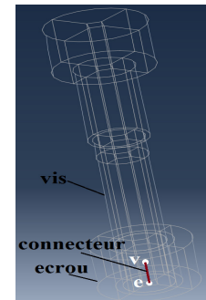
Figure 3. LIAISON PIVOT DANS LE BOULON
