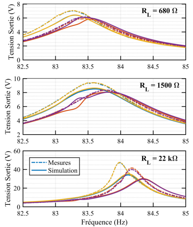
Fig. 13: Tensions de sortie obtenues expérimentalement et par simulation pour différentes résistances de charge R_L et pour V_{in} = 4 \text{ V}
