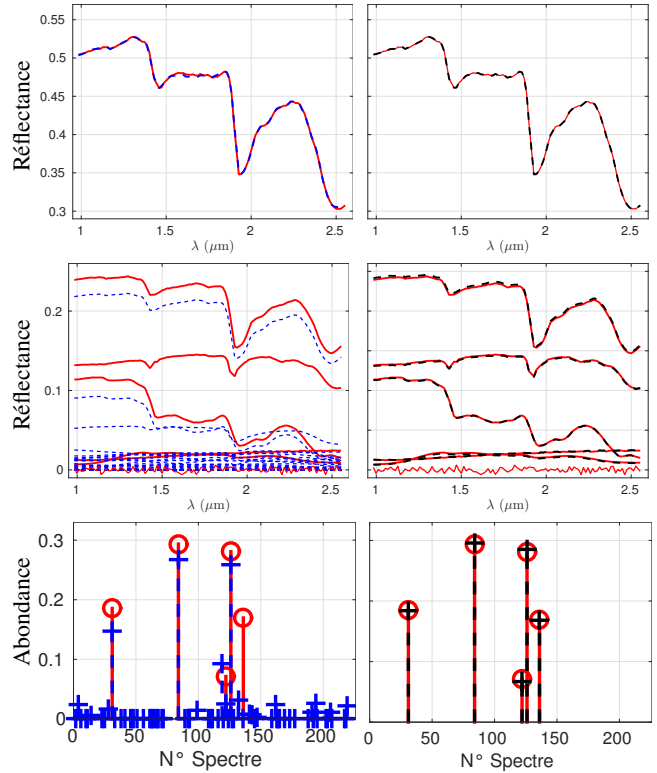
FIGURE 2 – Exemple de résultat ( K_{\max} = 5 spectres, RSB = 45 dB) : solution de FCLS (gauche) et solution exacte du problème \ell_0 (droite). En haut : spectre non bruité et sa reconstruction. Au centre, composantes estimées pondérées par les abondances (et bruit sur les données). En bas, abondances estimées. Les traits pleins rouges représentent les vraies valeurs et les pointillés leurs estimations.
