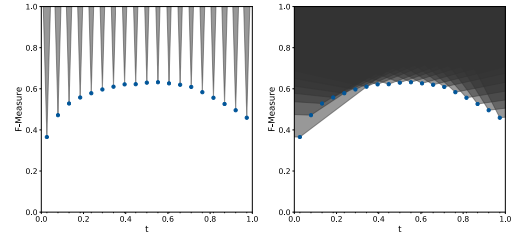
(d) IJCNN
