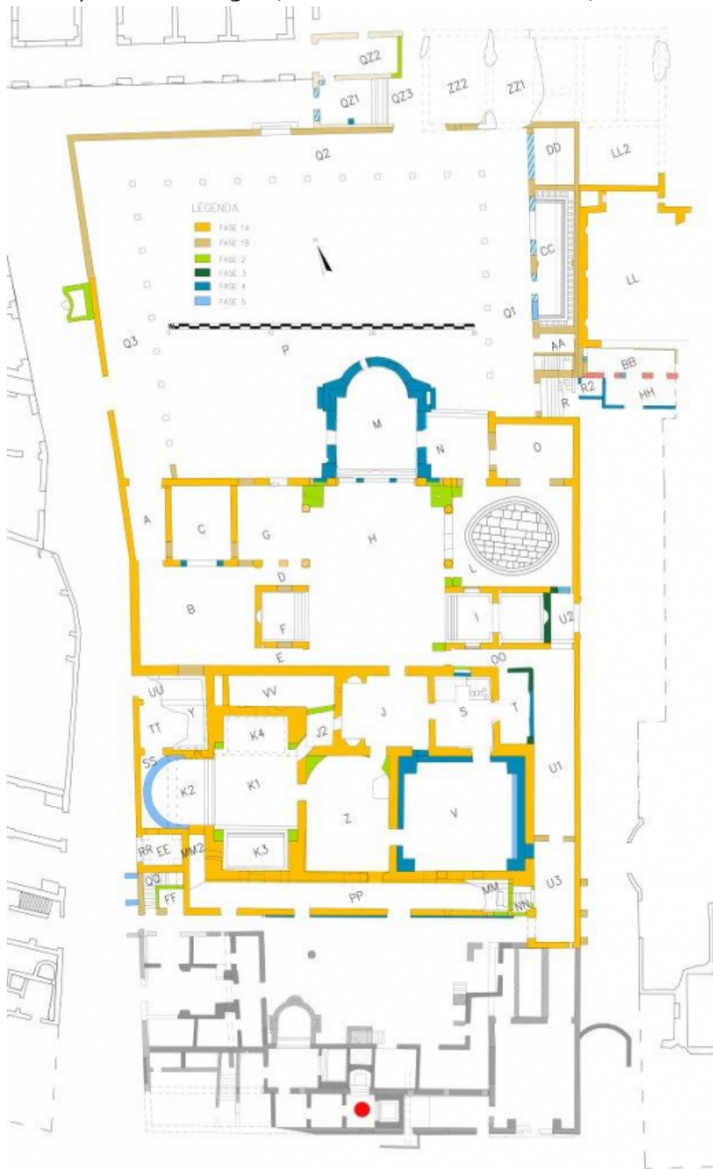
Fig. 2 – Le fasi edilizie delle Terme di Porta Marina. In rosso l'ambiente in cui venne rinvenuta l'epigrafe Ostia, inv. n. 11850 (elaborazione: M. Turci).
