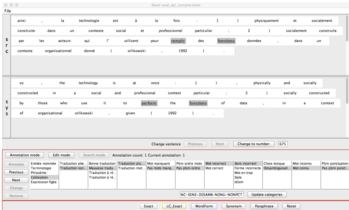
Figure 1 : Capture d'écran de l'outil Blast
