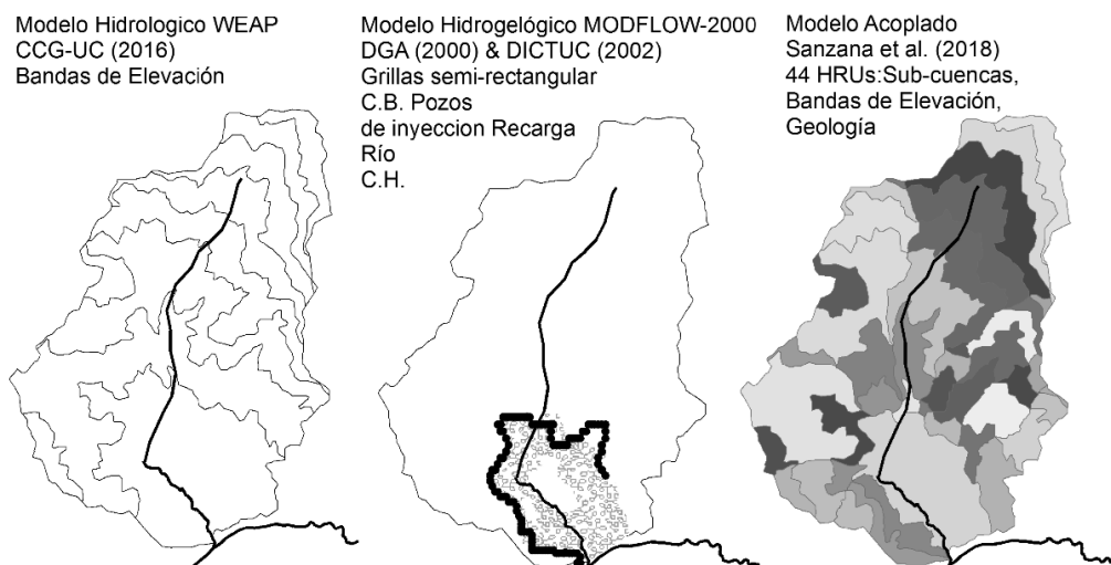
Figura 10.- Ejemplo de un esquema de preparación de segmentación espacial para el acople superficial y subterráneo
