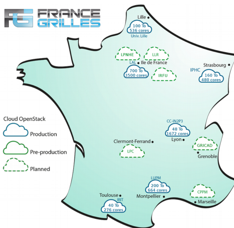
Figure 1 - Carte de France des sites participant à l'infrastructure
