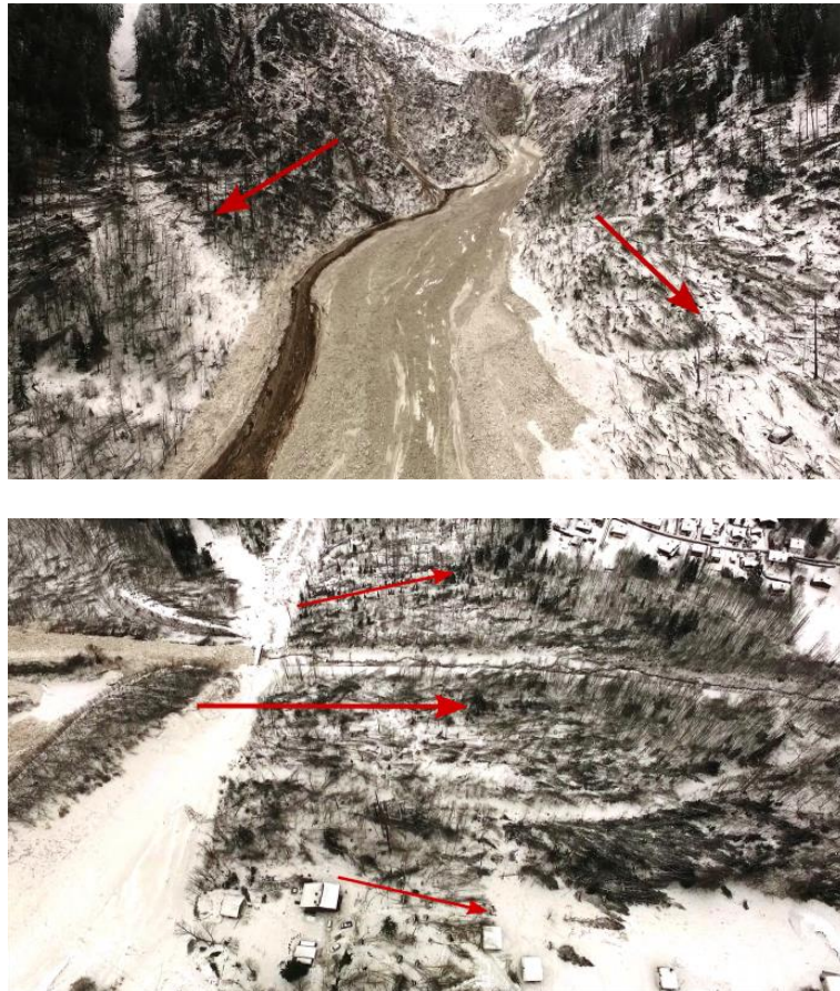
Figure 2. Exemples de dégâts causés par l'aérosol sur la forêt sur les rives droite et gauche en amont du paravalanche (photographie en haut ; ©Mairie de Chamonix) et au niveau des habitations en aval du paravalanche (photographie en bas ; ©Mairie de Chamonix). Les flèches en rouge indiquent les directions principales de l'aérosol.
