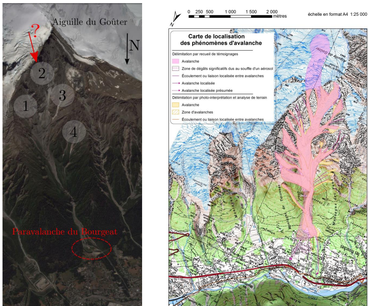
Figure 1. Vue générale du couloir d'avalanche du Bourgeat avec les principales zones de départ (photographie à gauche ; ©Google Earth), le paravalanche et les enjeux en aval du paravalanche. Emprises CLPA (édition 2004 avant révision suite à l'événement du 9 janvier 2018) du couloir du Bourgeat sur fond topographique IGN, montrant en particulier le fonctionnement de la liaison entre le couloir de Tacconnaz et celui du Bourgeat (image à droite).
