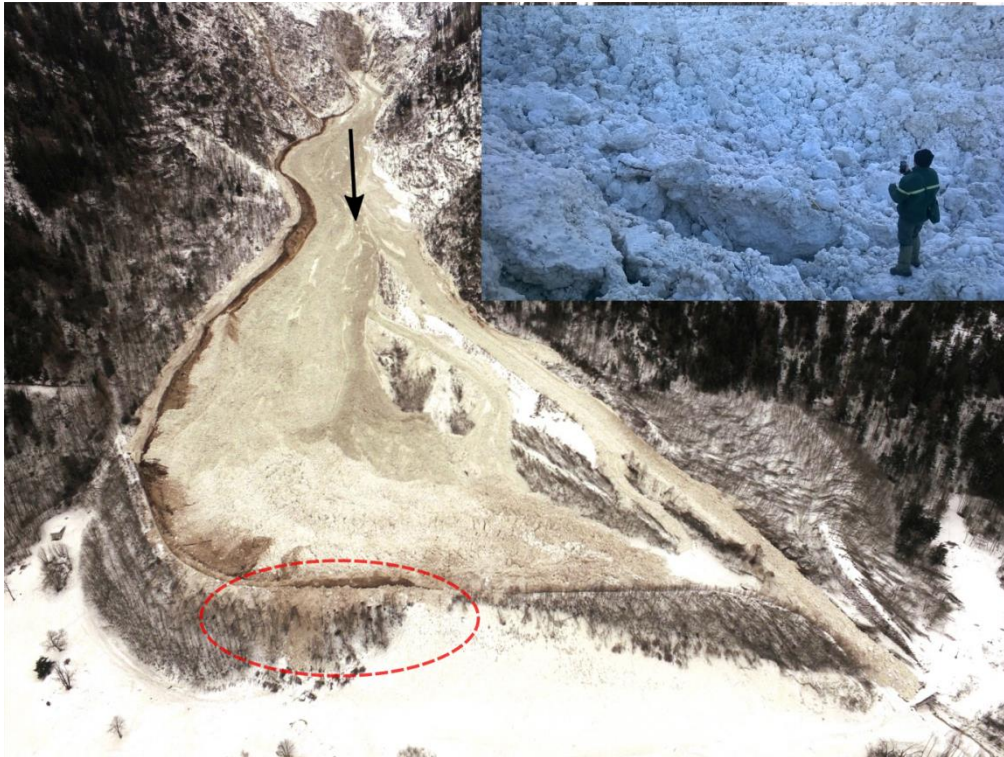
Figure 3. Dépôt de l'avalanche dans le paravalanche du Bourgeat (@Mairie de Chamonix). L'ellipse tracée en pointillé rouge montre la zone des débordements mineurs, là où une langue d'avalanche s'est propagée le long de la digue avec une hauteur supérieure à la digue. L'image insérée (@Irstea-Thierry Faug) montre un zoom du dépôt illustrant ainsi le caractère granulaire de ce dépôt et la taille importante de certains agrégats de neige (à comparer à l'échelle donnée par la personne).
