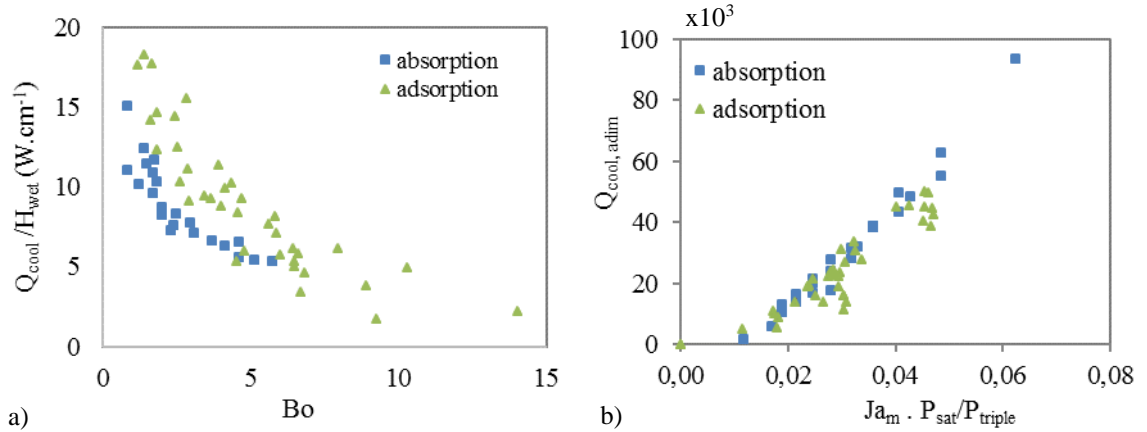
Figure 6 : Evolution de a) la puissance spécifique en fonction du nombre de Bond b) d'une puissance frigorifique adimensionnelle en fonction du produit du nombre de Jakob par le ratio P_{sat}/P_{triple}
